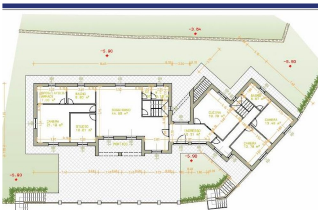
PIANTA PIANO TERRENO - scala 1:10
